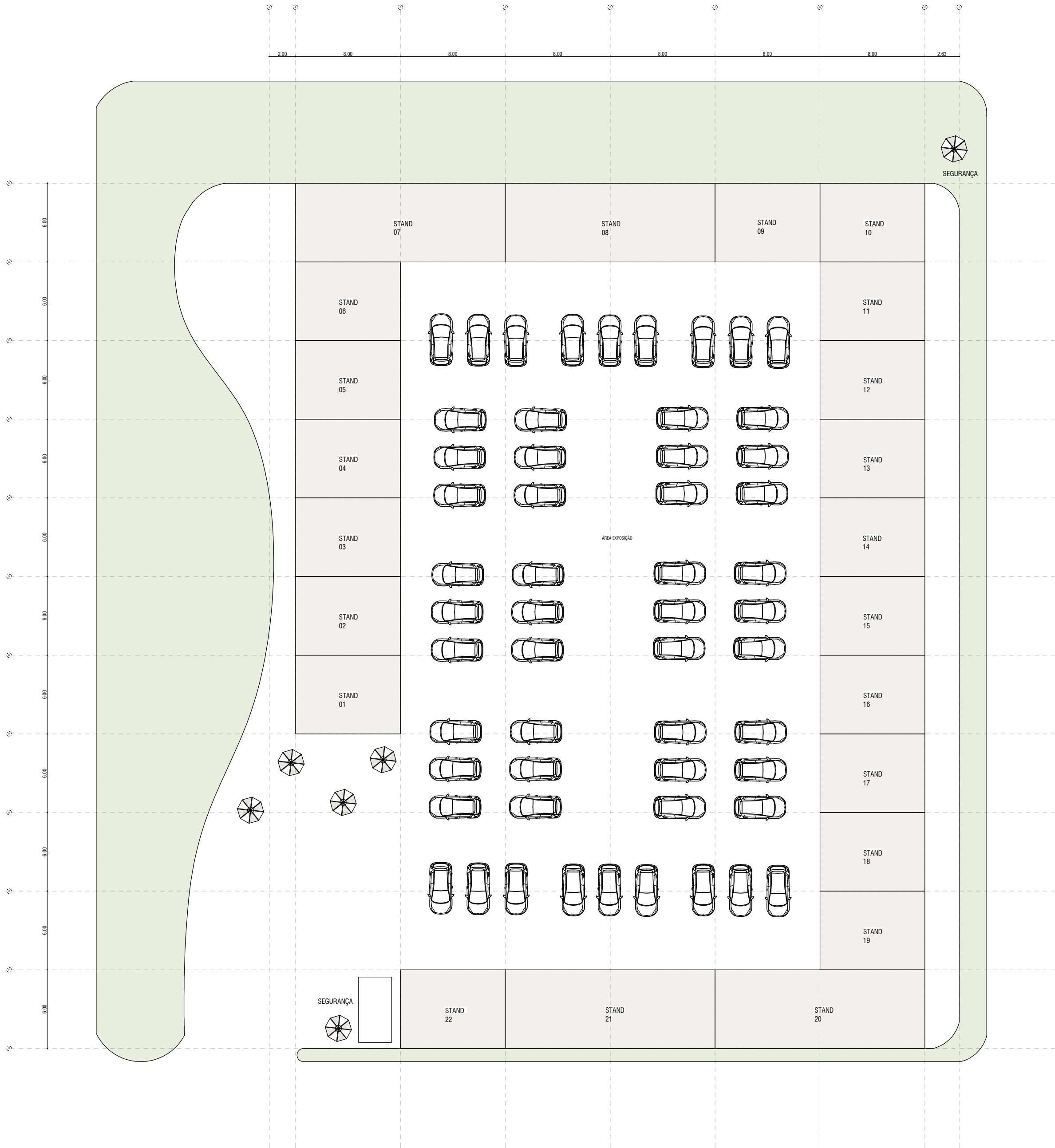
IMPLANTAÇÃO ESCALA 1:100
